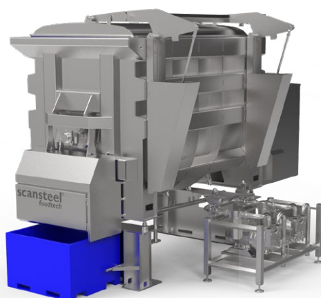
scanDefrost 9000 L.
